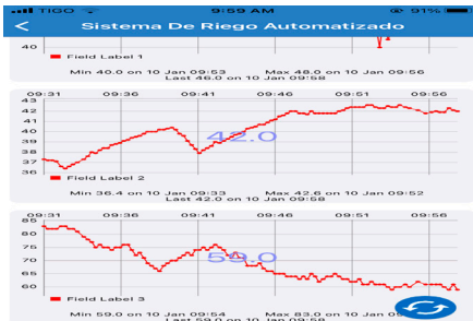
Fig. 8 Sensor de humedad del sustrato
