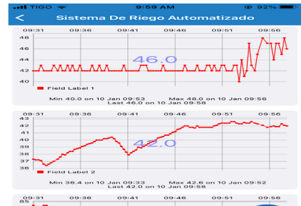
Fig. 10 Sensor de temperatura
