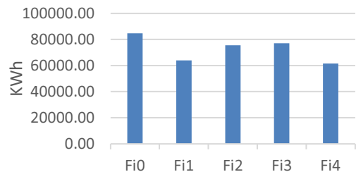
Figura 10. Ganancias solares por paredes edificio de oficinas.
