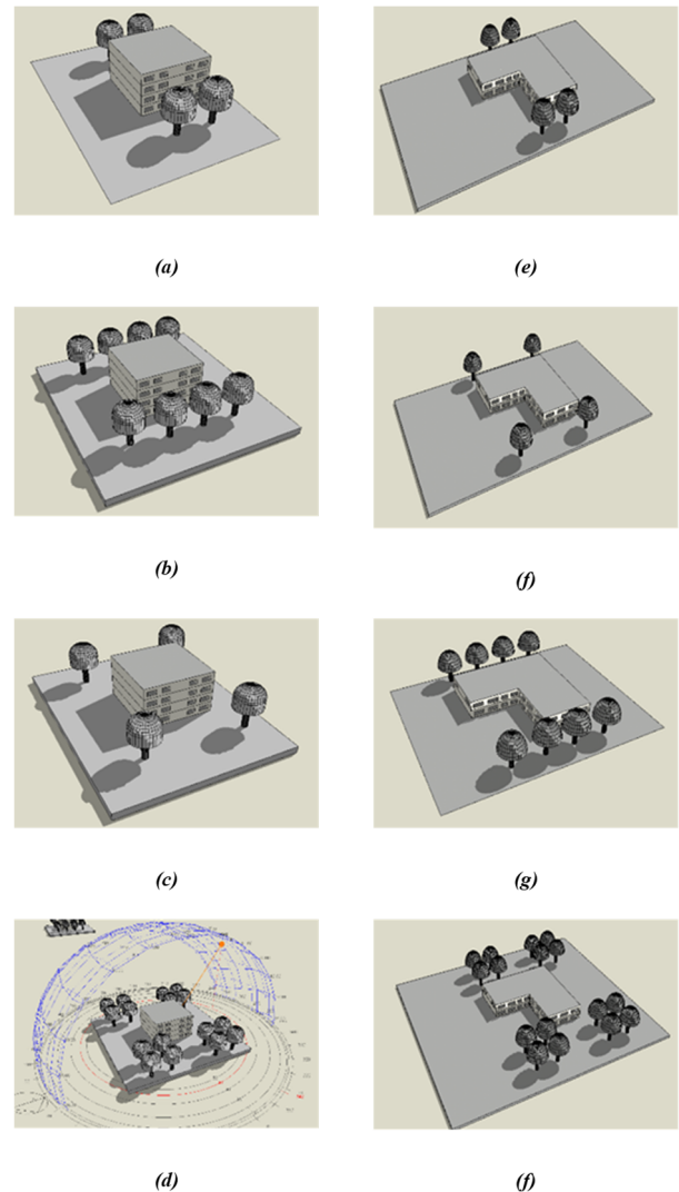
Figura 4. Escenarios de arborización para los edificios: (a)-Fi1 edificio de apartamento, (b)- Fi2 edificio de apartamentos, (c)-Fi3 edificio de apartamentos, (d)-Fi4 edificio de apartamentos, (e)-Fi1 edificio de oficina, (f)-Fi3 edificio de oficina, (g)-Fi2 edificio de oficina, (h)-Fi4 edificio de oficina. De arriba hacia abajo los Fi son: Fi1, Fi2, Fi3, Fi4 (11.05, 5.53, 15.64, 3.9).
