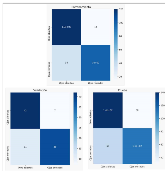
Figura 6. Matrices de confusión para conjunto de entrenamiento, validación y pruebas.
