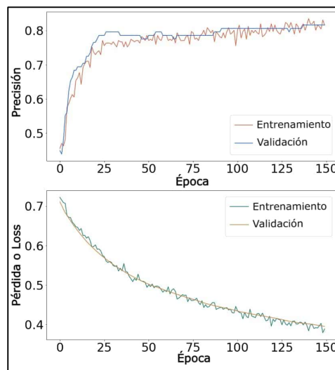
Figura 5. Gráfica de precisión y valor de pérdida para datos de entrenamiento y validación.
