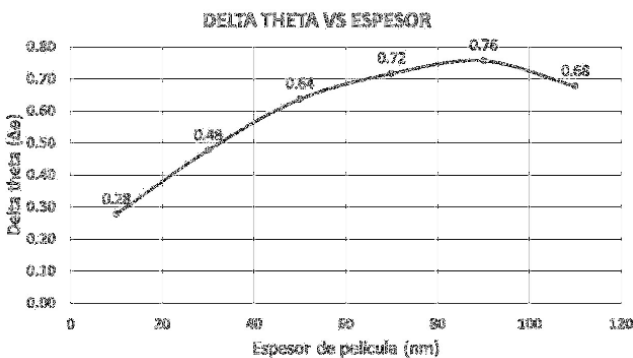
Figura 4. Variación del ángulo de incidencia (Delta theta) vs el Espesor de película delgada de oro.
