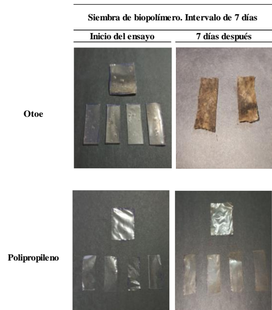
Figura 11 ensayo de biodegradación mediante siembra. Intervalo de 7 días con biopolímero de oteo y polipropileno.
