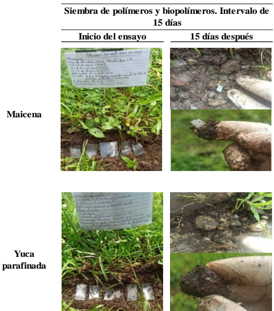
Figura 12 ensayo de biodegradación mediante siembra. Intervalo de 15 días con biopolímero de maicena y yuca.
