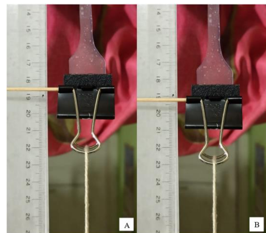
Figura 4. Posición inicial de una probeta de yuca (A) y posición final de la misma probeta antes de la fractura (B).
