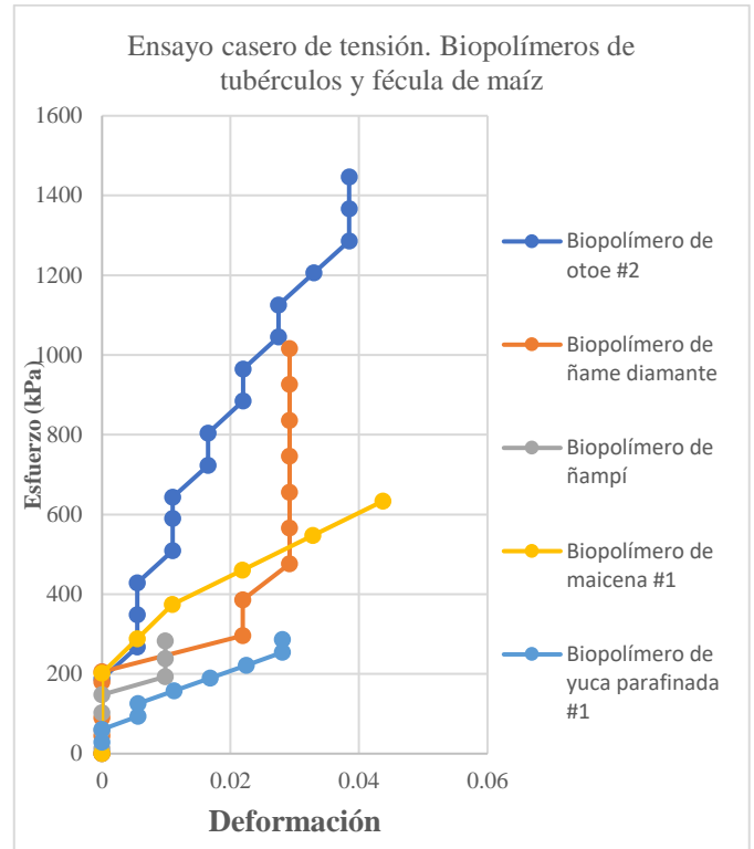
Gráfica 1 Ensayo casero de tensión de probetas de biopolímeros compilados y probeta de maicena.
