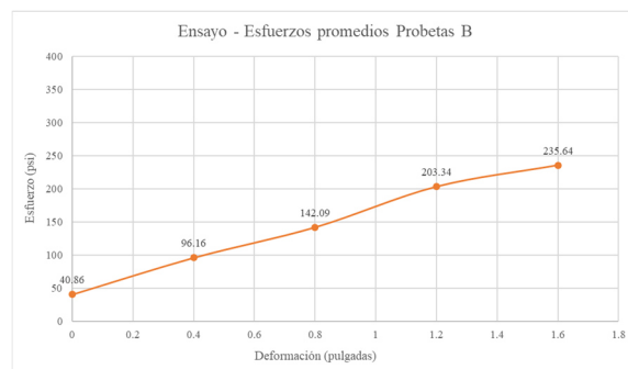
Figura 6. Esfuerzo vs deformación del promedio obtenido con las probetas B.
