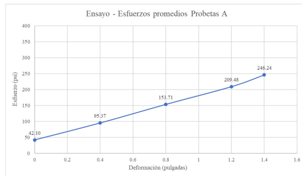
Figura 5. Esfuerzo vs deformación del promedio obtenido con las probetas A.
