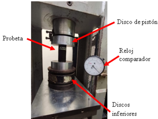
Figura 2. Probeta A1 lista para ser ensayada.
