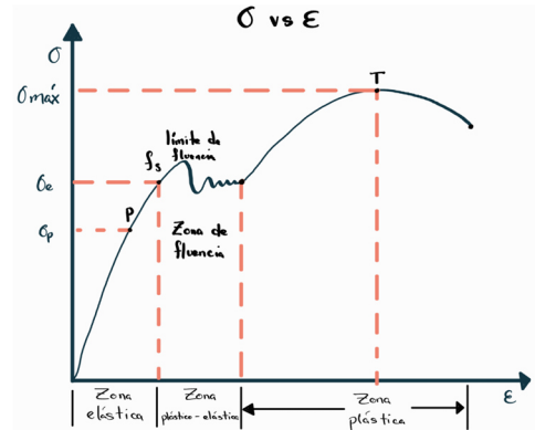
Figura 3. Gráfica esfuerzo vs deformación típica de materiales [6].
