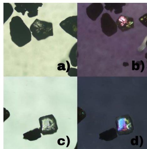
Figura 3. a) Mineral piroxeno en nicols paralelo con objetivo 4x/0.1, b) mineral de piroxeno vista a nicols cruzados con objetivo 4x/0.1, c) mineral de olivino vista a nicols cruzados con objetivo 4x/0.1, d) mineral de olivino vista a nicols cruzados con objetivo 4x/0.1.
