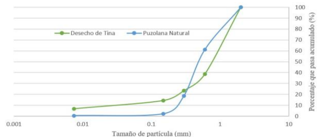
Figura 2. Distribución granulométrica.
