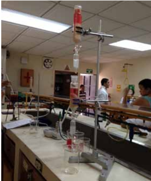
Figura 6. Disposición de biofiltros en serie para el tratamiento de efluentes con pigmentos orgánicos de origen animal.
